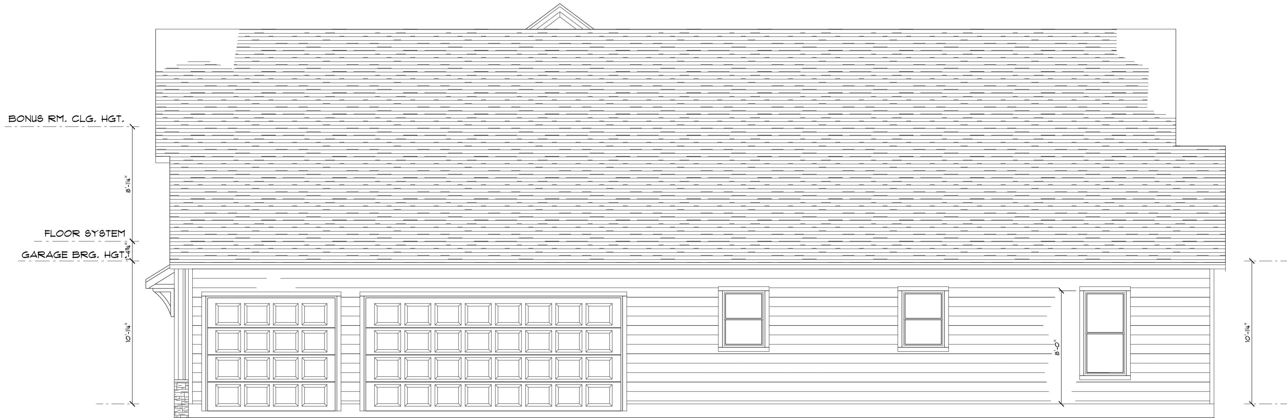
RIGHT ELEVATION
